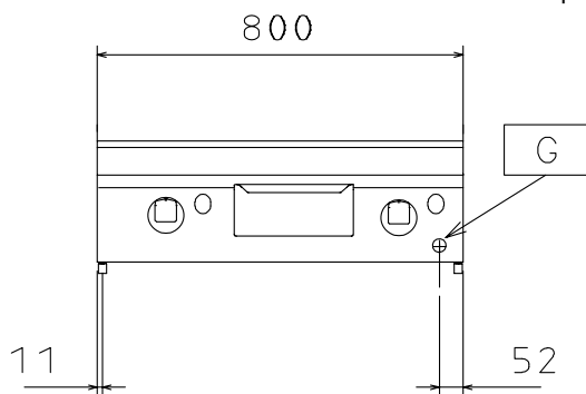
Zepředu
